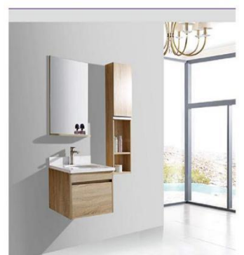
KA-GZ1042 Cabinet 主柜 580*530*400mm Mirror 镜子 550*140*750mm Side cabinet 侧柜 320*190*1200mm Countertop 台面 600*540mm
